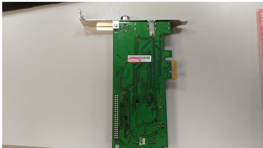
A757 AVerTV Nova T2
